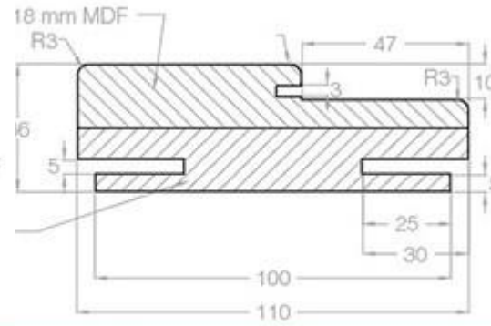
36 mm Kaplamalı Sandviç Kasa
