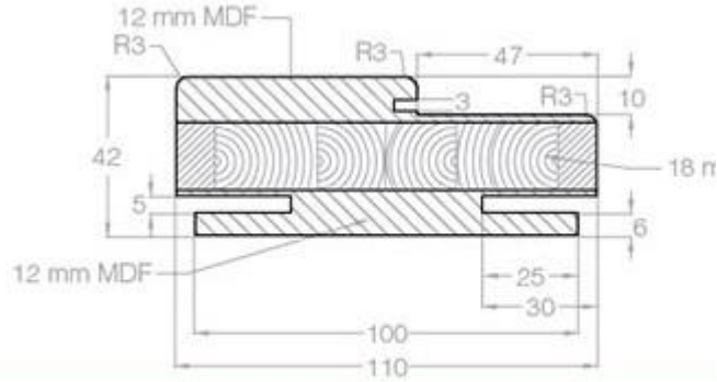
42 mm Kaplamalı Sandviç Kasa
