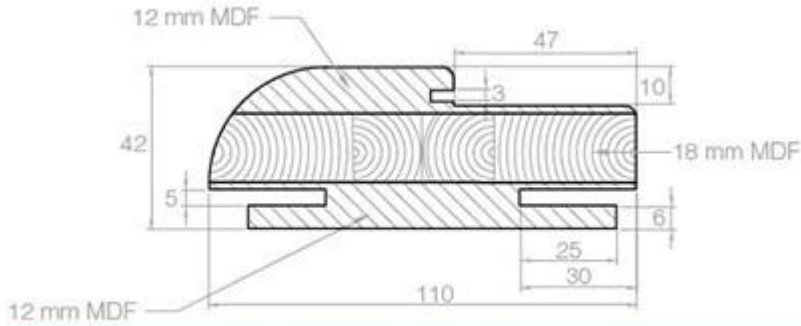
42 mm Bombeli Sandviç Kasa
