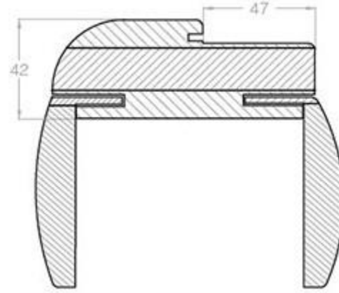
42 mm Kasa ve Pervaz Detayı
